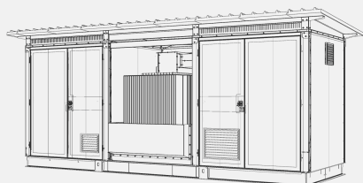
Espe Power Skid con trasformatore in olio
