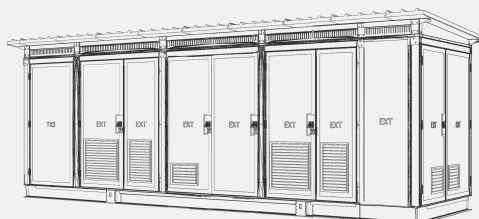
Espe Power Shelter (versione doppia) con doppio trasformatore in resina
